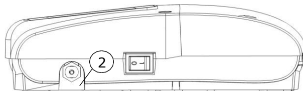
Перезагрузка ограничителя температуры STB: 1 – крышка-колпачок, 2 – кнопка перезагрузки.
